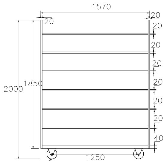
示范菌蛋集中出菇房灭菌车正立面图
