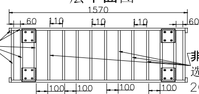
示范菌蛋集中出菇房灭菌车底层平面图
