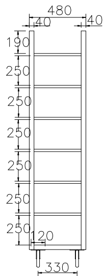
示范菌蛋集中出菇房灭菌车侧立面图
